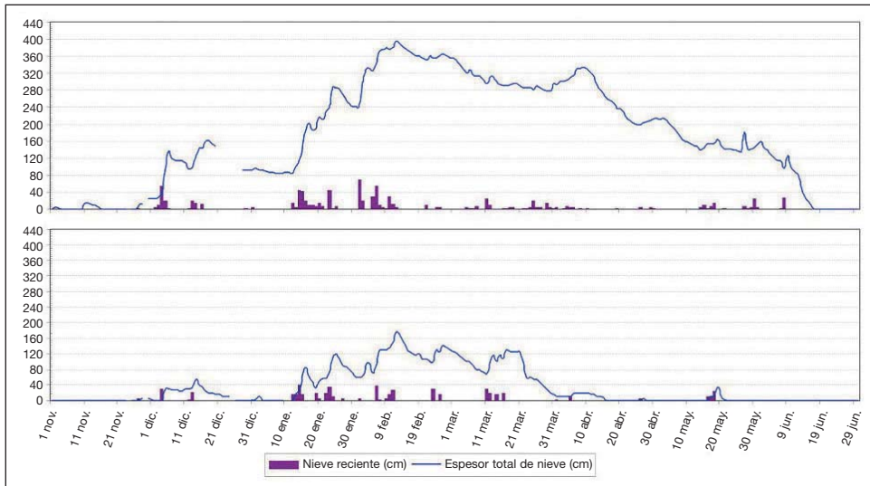
Fig. 3. Evolución del espesor total de nieve acumulado y nieve reciente en 24 horas durante la temporada invernal 2012-2013 en las estaciones de Resposuso (2200 m) (gráfico superior) y Lizara (1540 m) (gráfico inferior).
