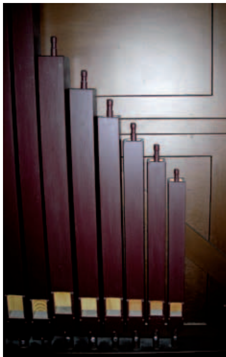
Pedalero y tubos del pedal de bordón 16'.
